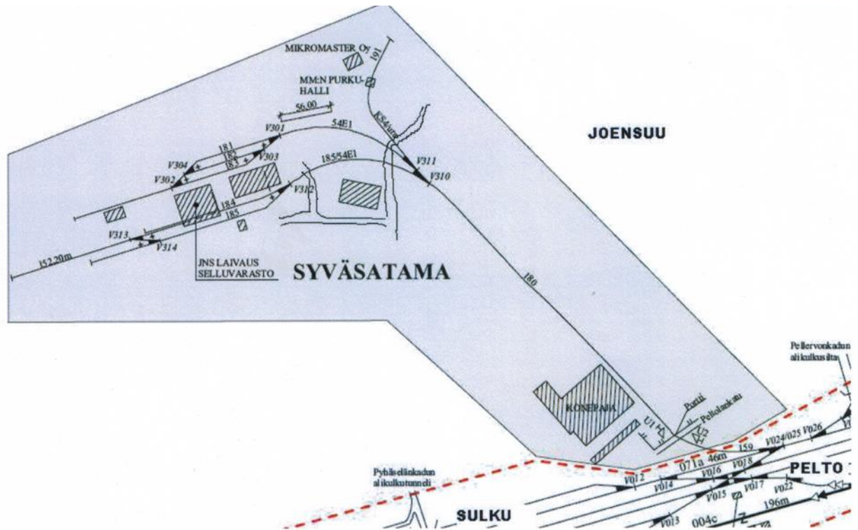
Kuva 1 Raiteistokaavio
